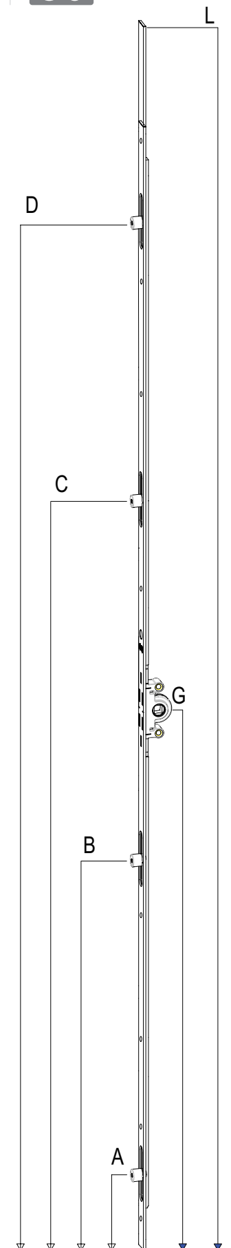
Asta a rulli per apertura a bandiera- Mantellina ad altezza costante
